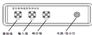
图 1a 变压器绕组变形测试仪前面板图(前面板)
