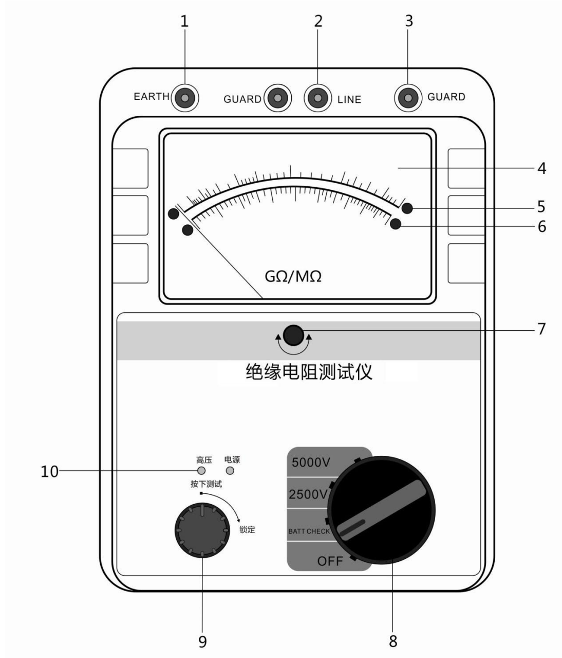
图 1：结构图
